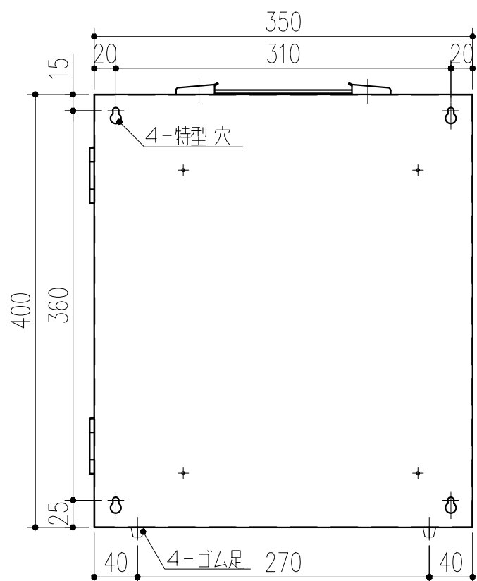
背面図 S=1/5
