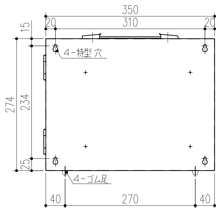
背面図 S=1/5
