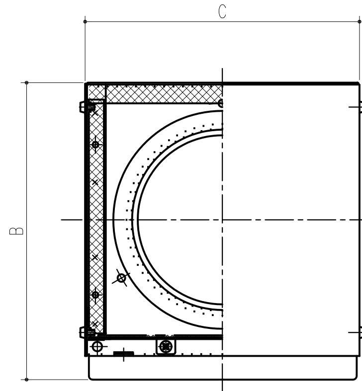
X-X矢視図
