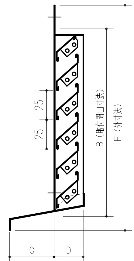
縦断面図
