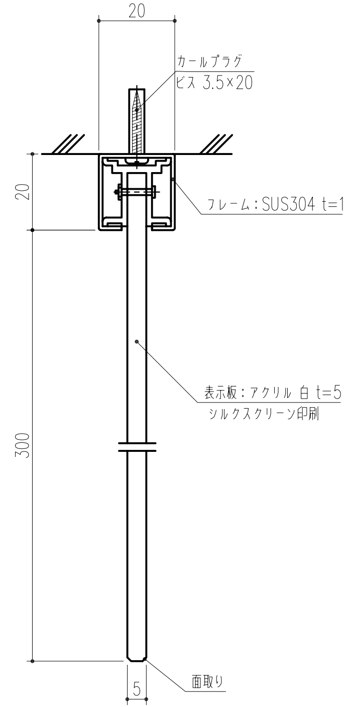
横断面図 s=1/1
