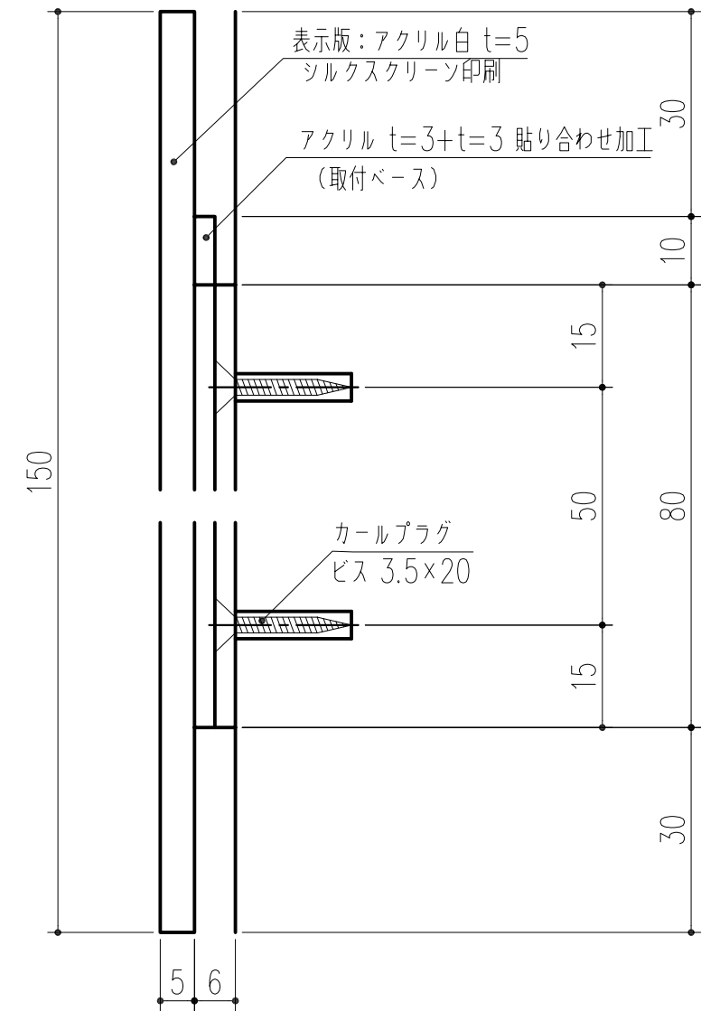
縦断面図 s=1/1
