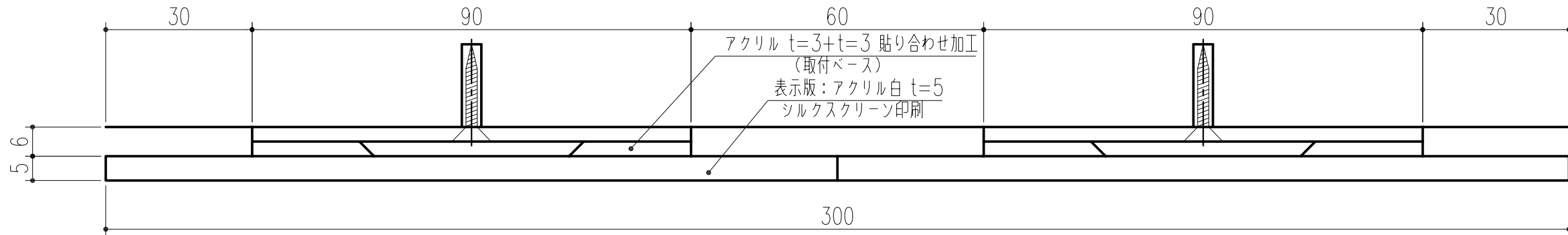
横断面図 s=1/1
