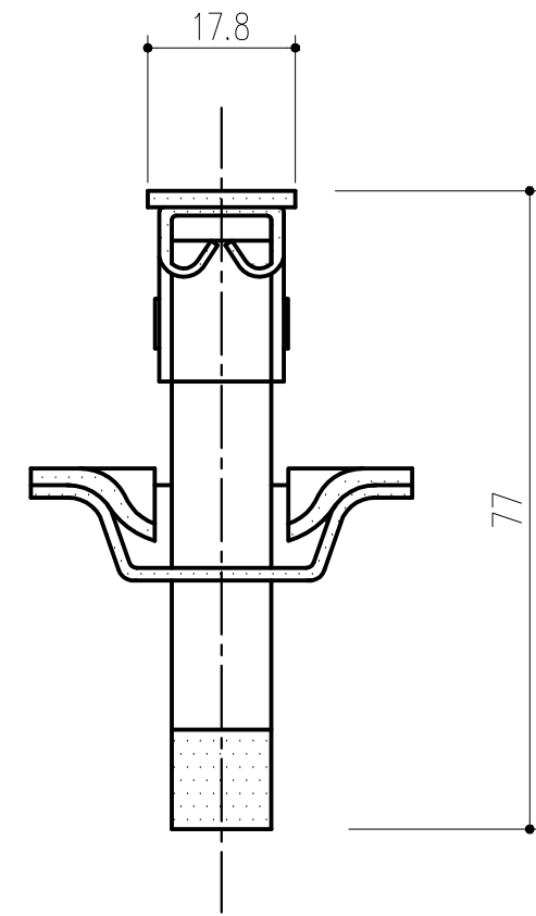
A-A'断面図 ●床開口寸法 126×34 本製品は改良の為予告なしに変更する事があります。
