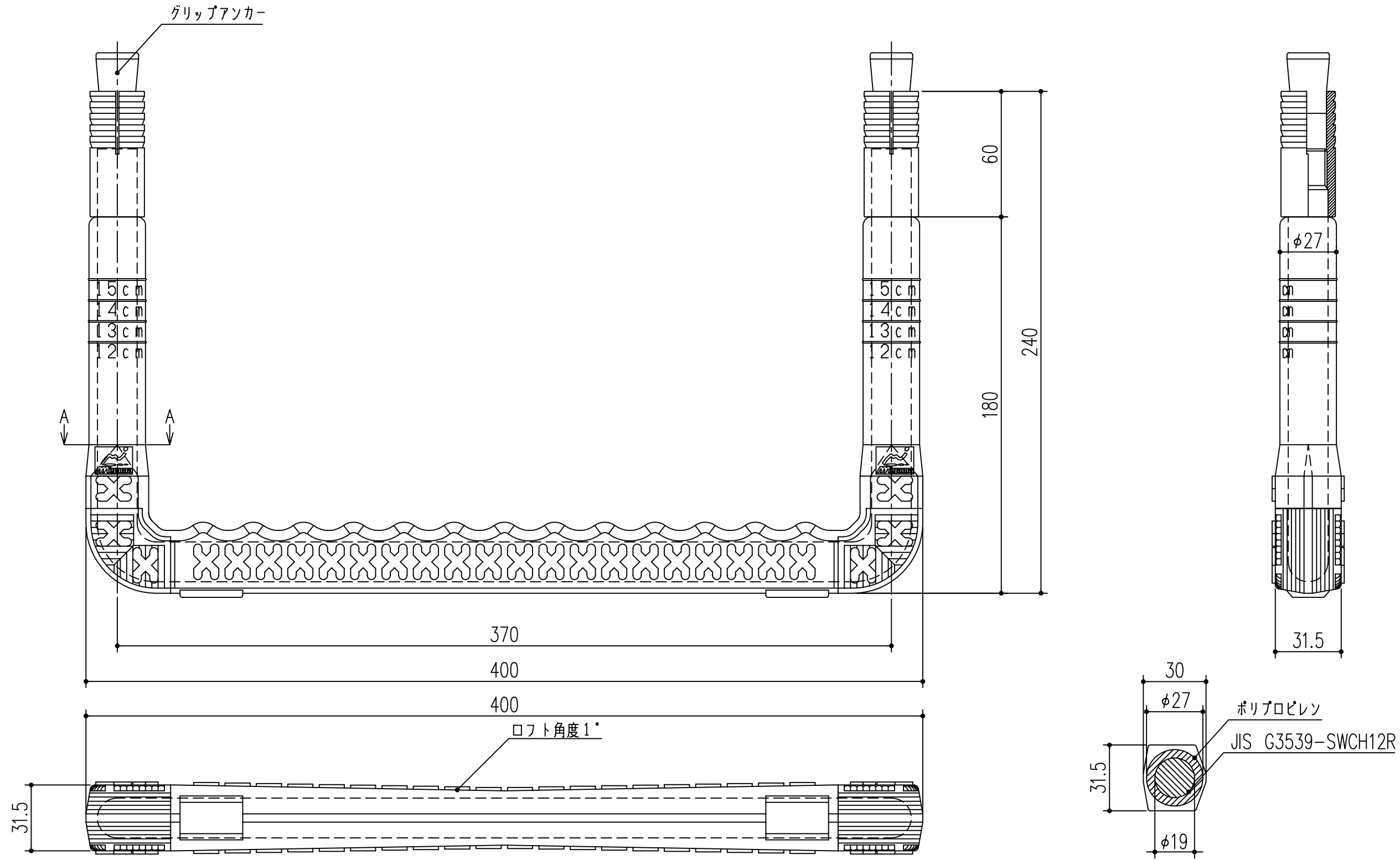
A-A断面図
