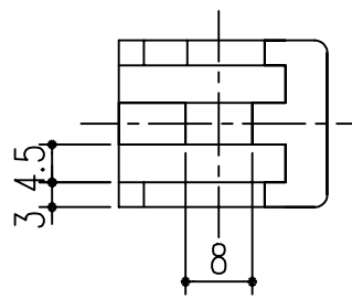
A-A' 断面
