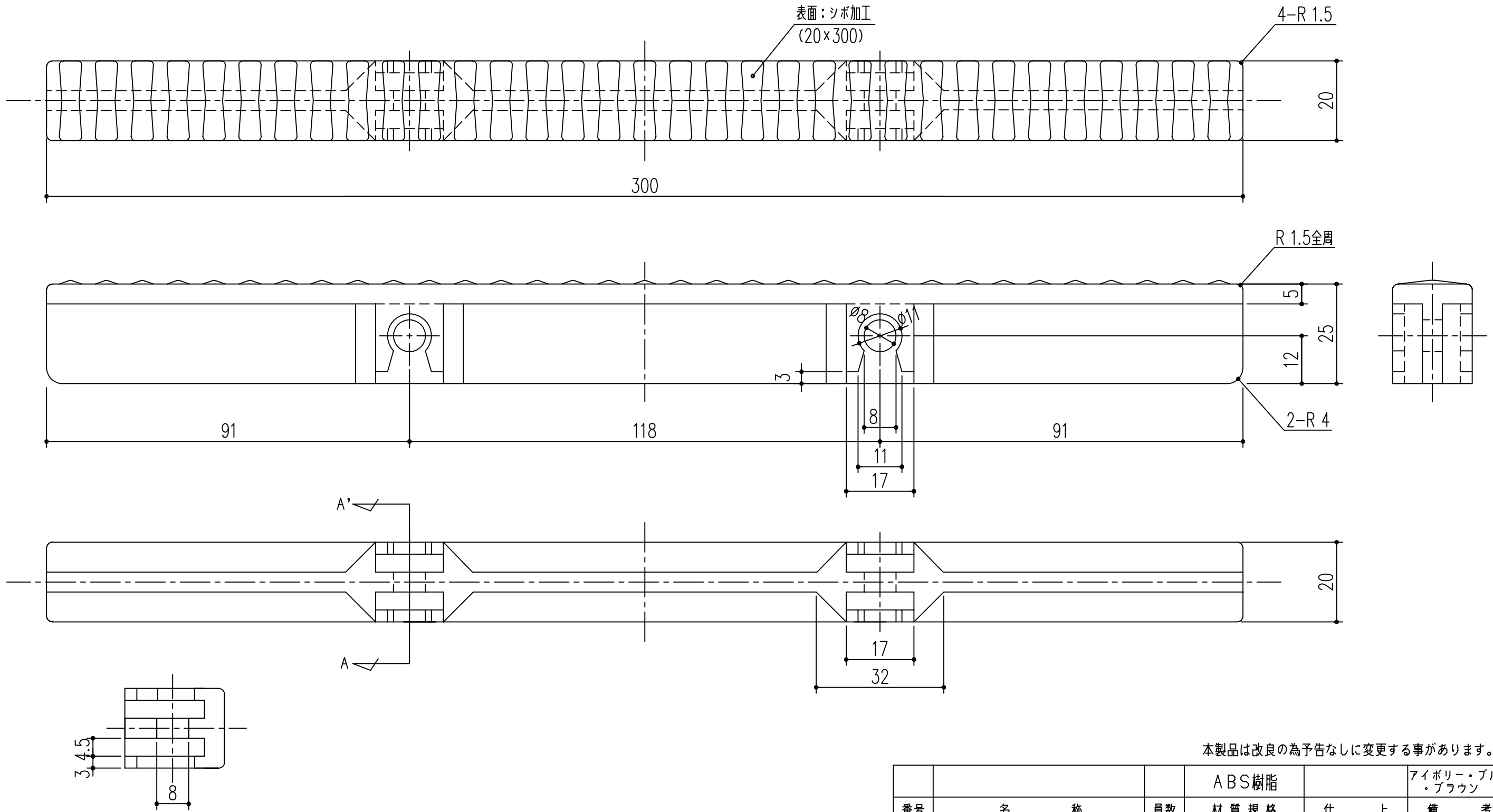
A-A' 断面
