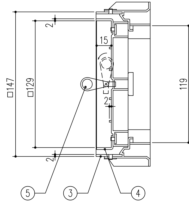
A-A'断面図
