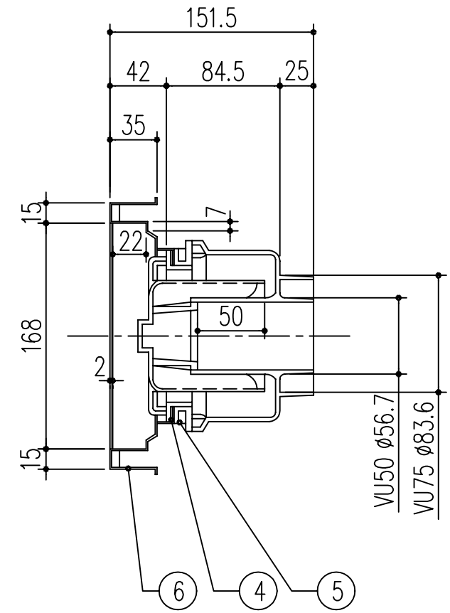
A-A'断面図
