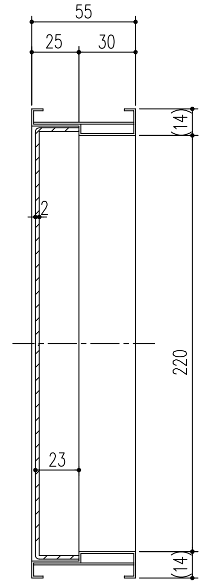
A-A' 断面図
