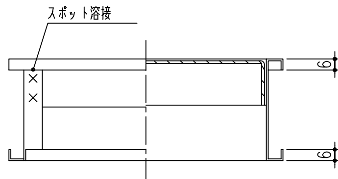
B-B' 矢視
