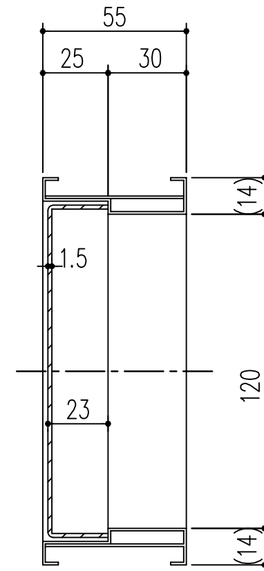
A-A' 断面図
