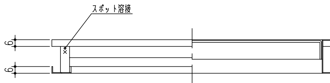
B-B' 矢視
