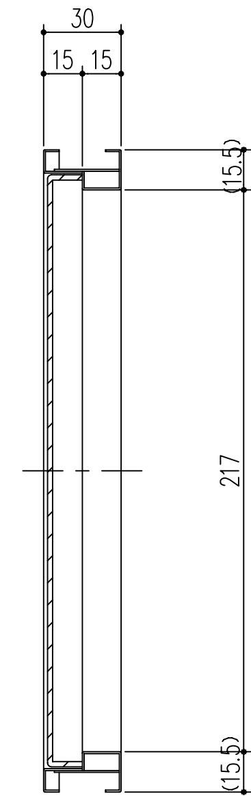
A-A' 断面図
