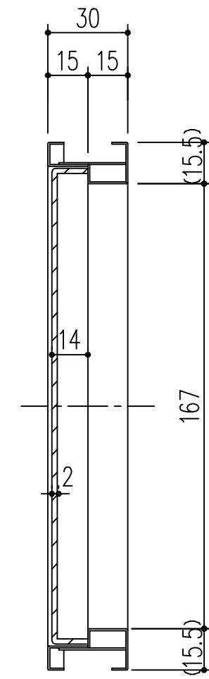
A-A' 断面図
