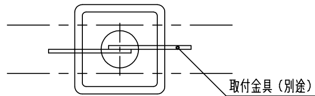
クサリ縦といの取付け例
