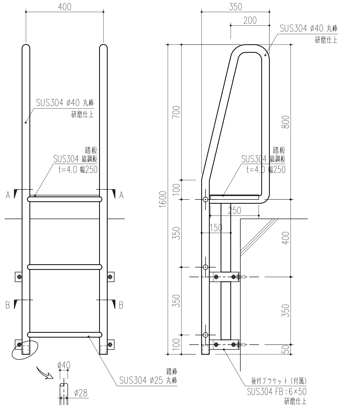
姿図 S=1:10
