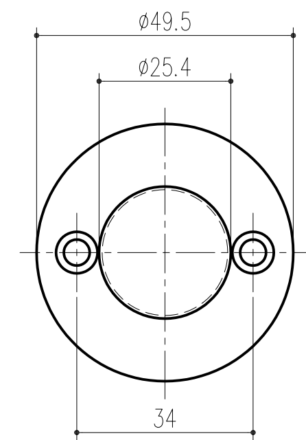
取付丸座 1/1
