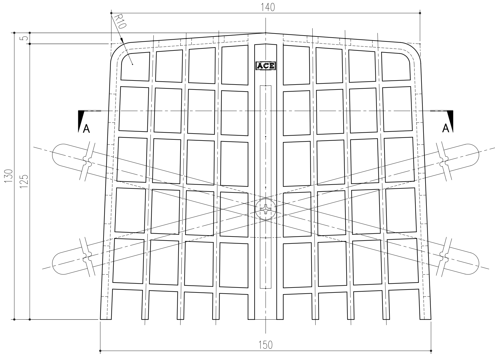
外観(正面)図
