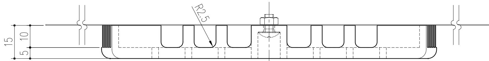
上面図
