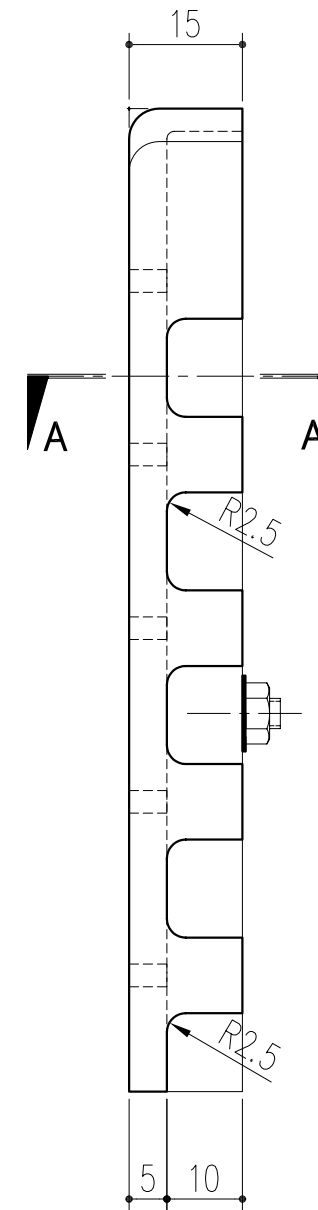
側面図
