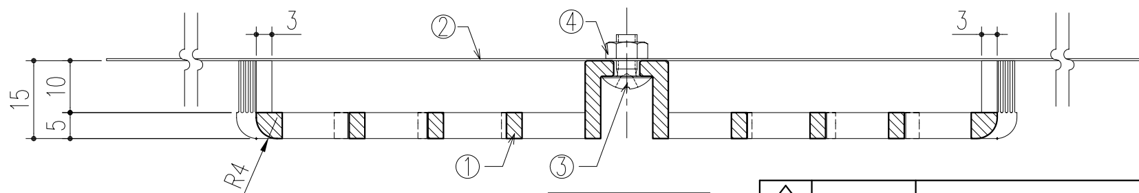
A-A断面図
