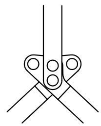
SUパイプ使用時の穴セット例
