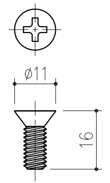
SUS十字穴付皿小ネジ M6×16
