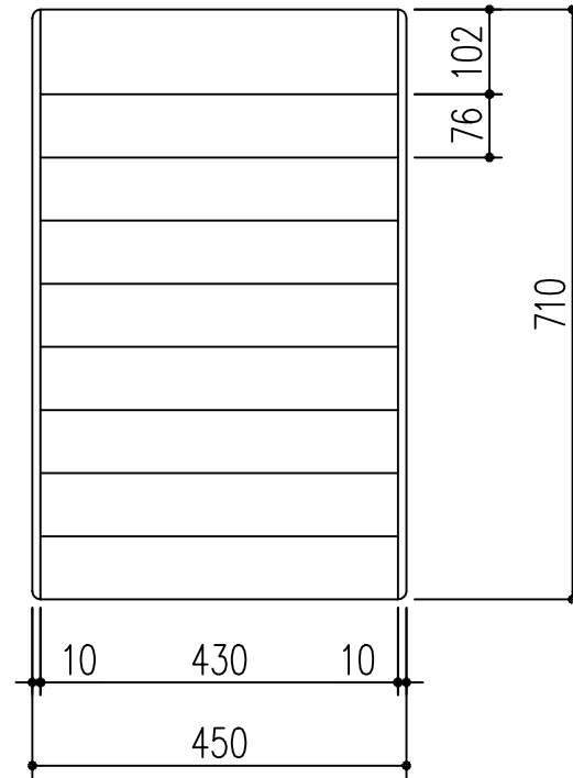
SYD-03L h=102 (1段) + 76 (8段)
