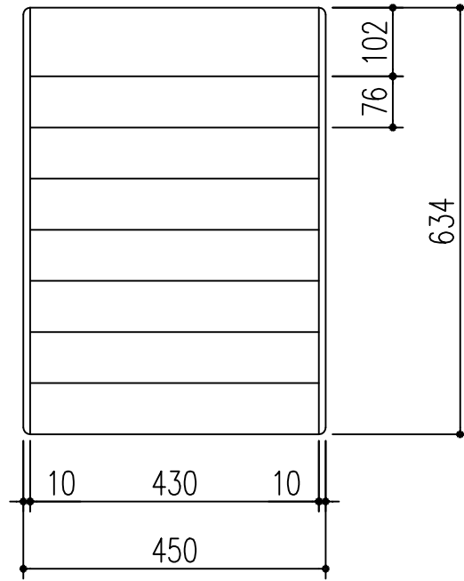
SYD-02L h=102 (1段) + 76 (7段)
