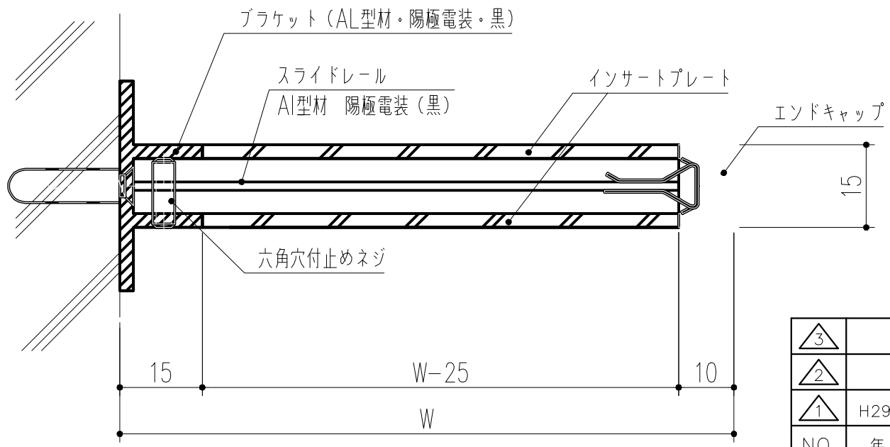
突出し (S=1/1)
