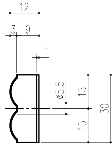
A-A 断面 S=1/1
