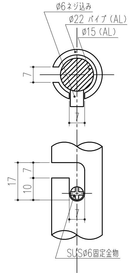
A部詳細図 S=1/1
