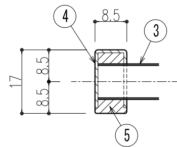
B-B断面図 S=1:1
