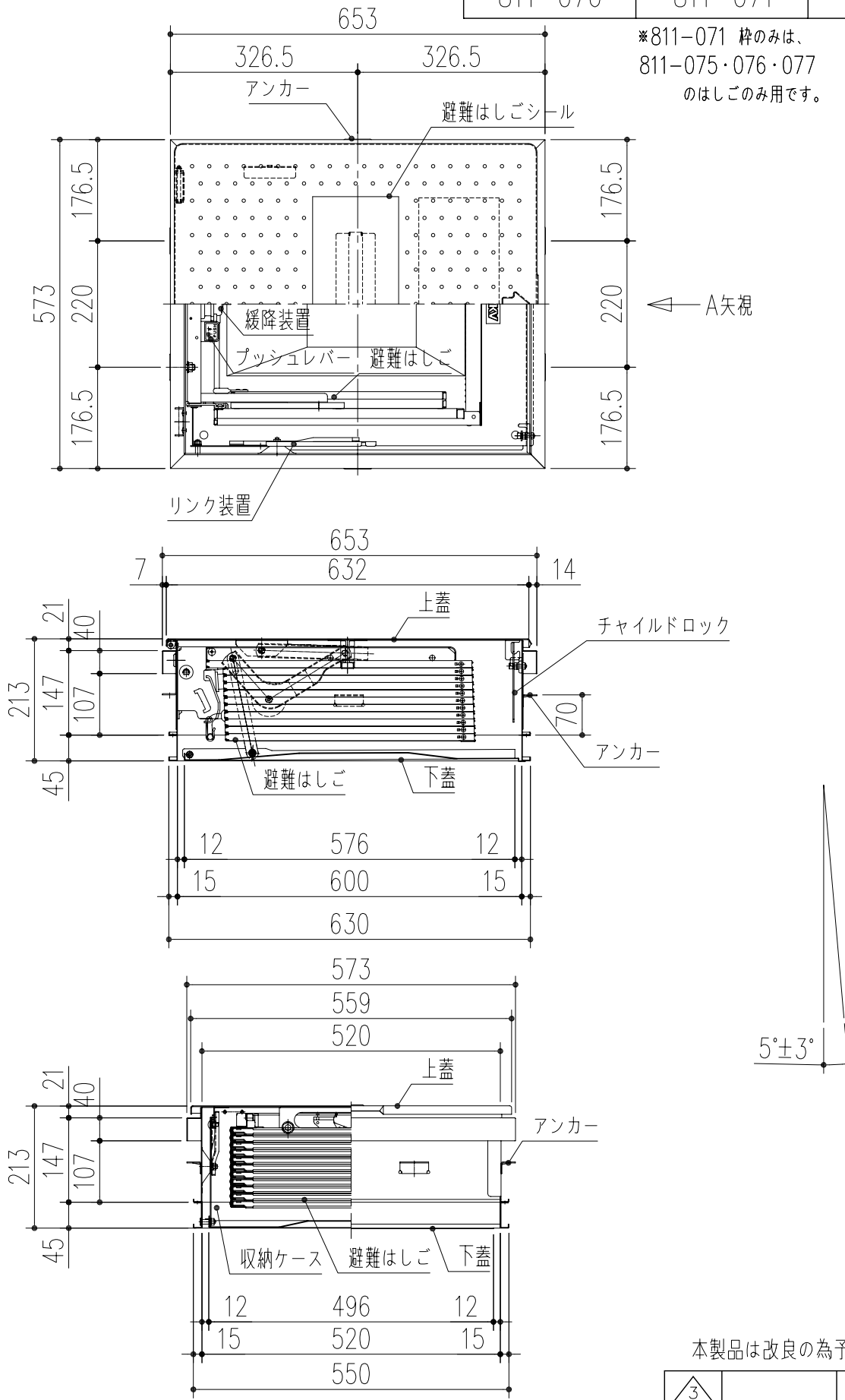
A矢視図 収納状態 S=1/10
