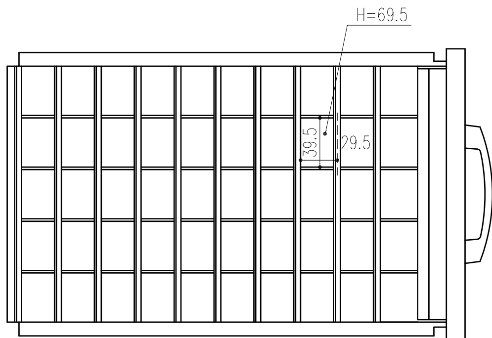
引出し平面図
