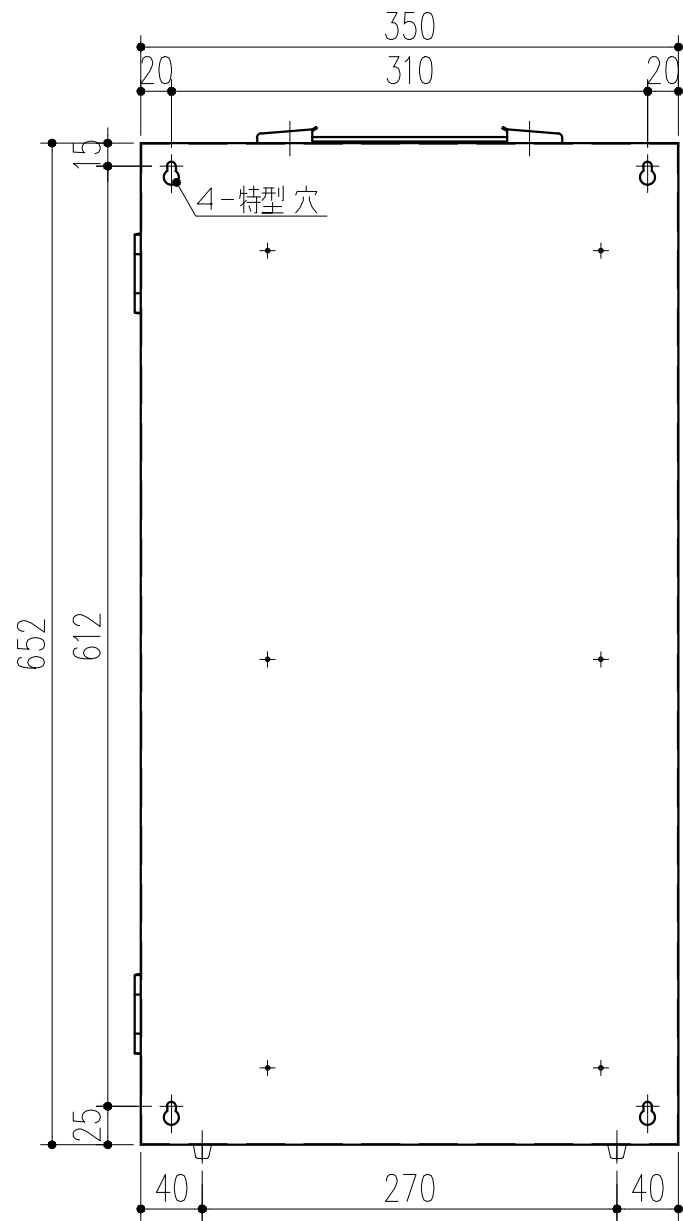
背面図 S=1/5
