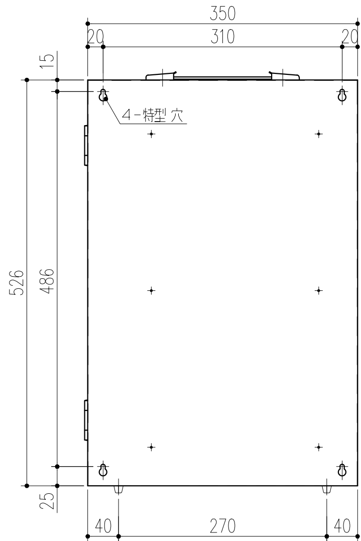
背面図 S=1/5
