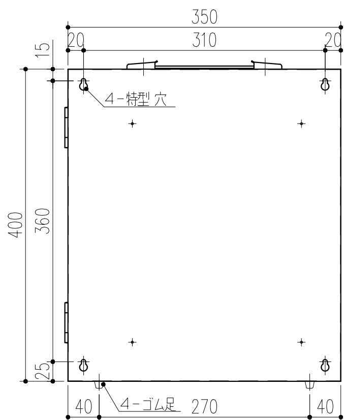
背面図 S=1/5
