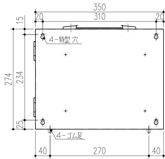
背面図 S=1/5
