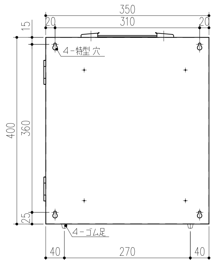
背面図 S=1/5
