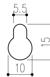
壁掛け用ビス穴 詳細図 S=1/1
