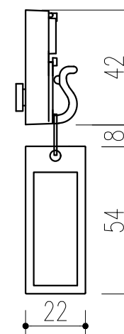
キーホルダー 詳細図 S=1/2
