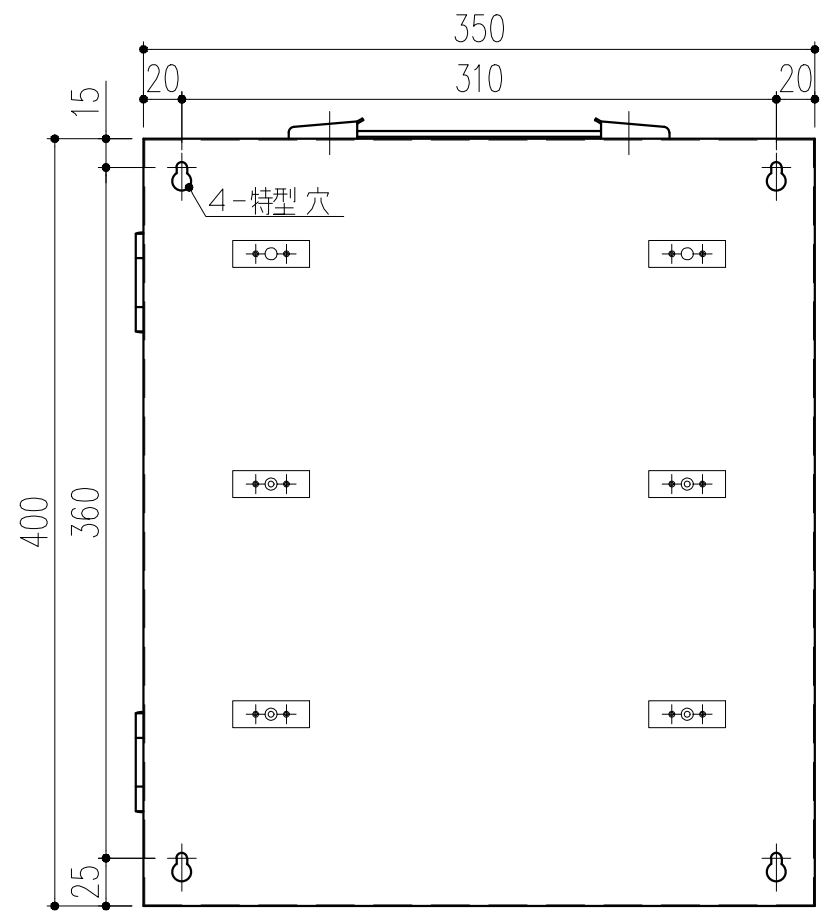
背面図 S=1/4
