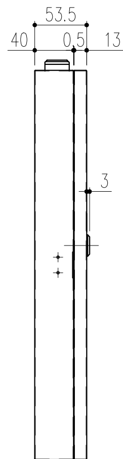
側面図 S=1/4
