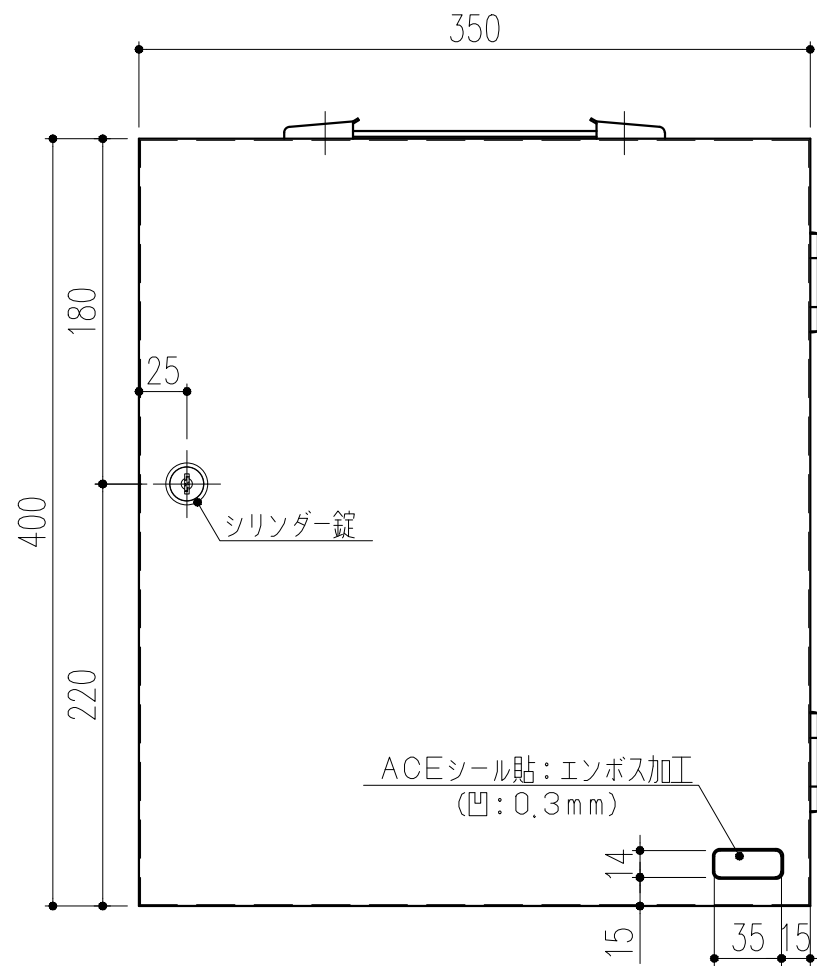
正面図 S=1/4
