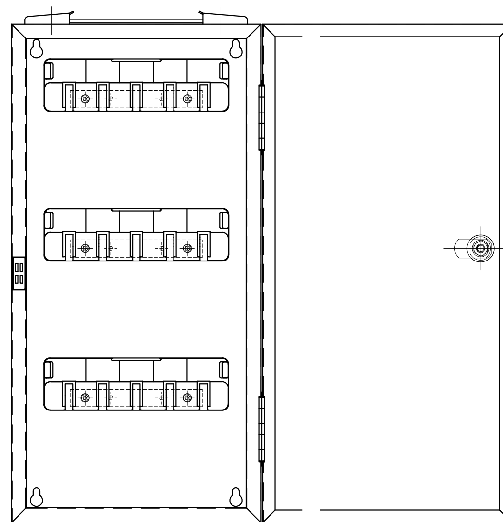
扉開放図 S=1/3
