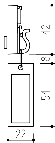
キーホルダー 詳細図 S=1/2
