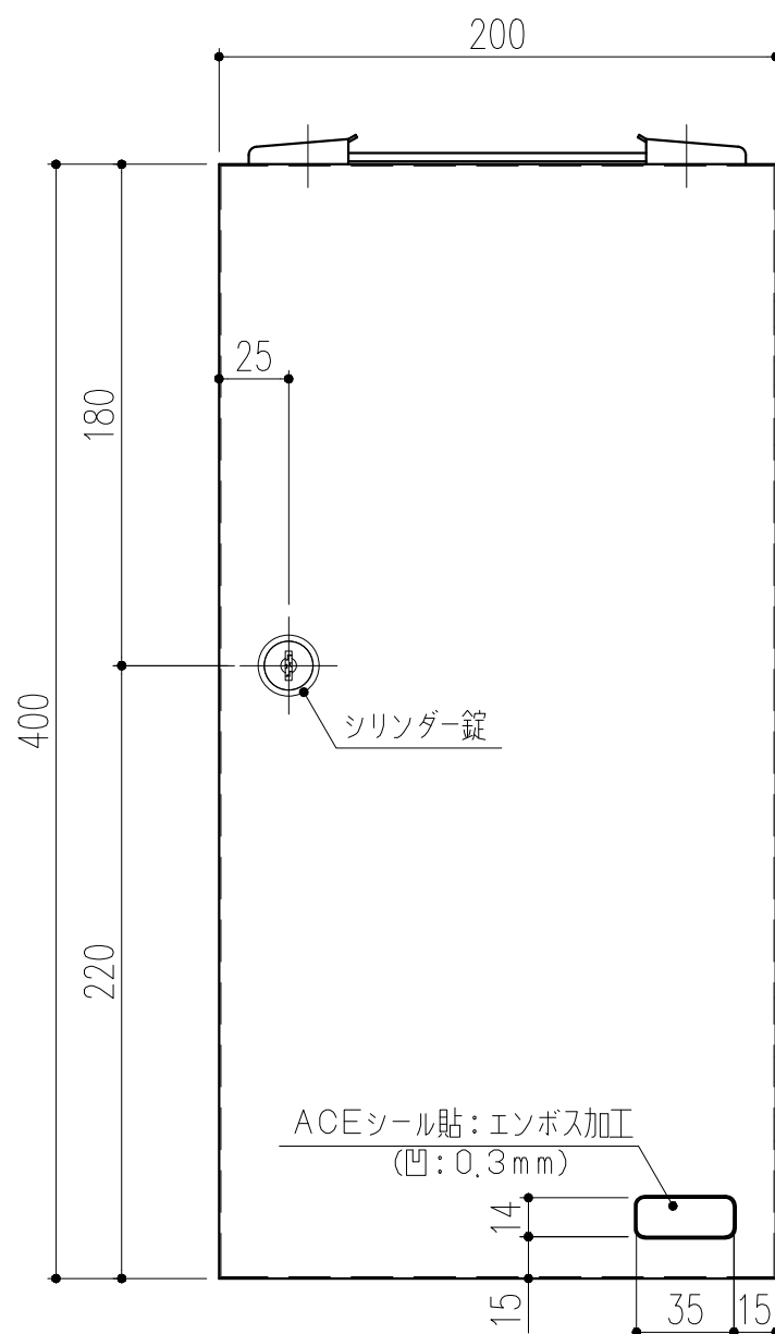
正面図 S=1/3
