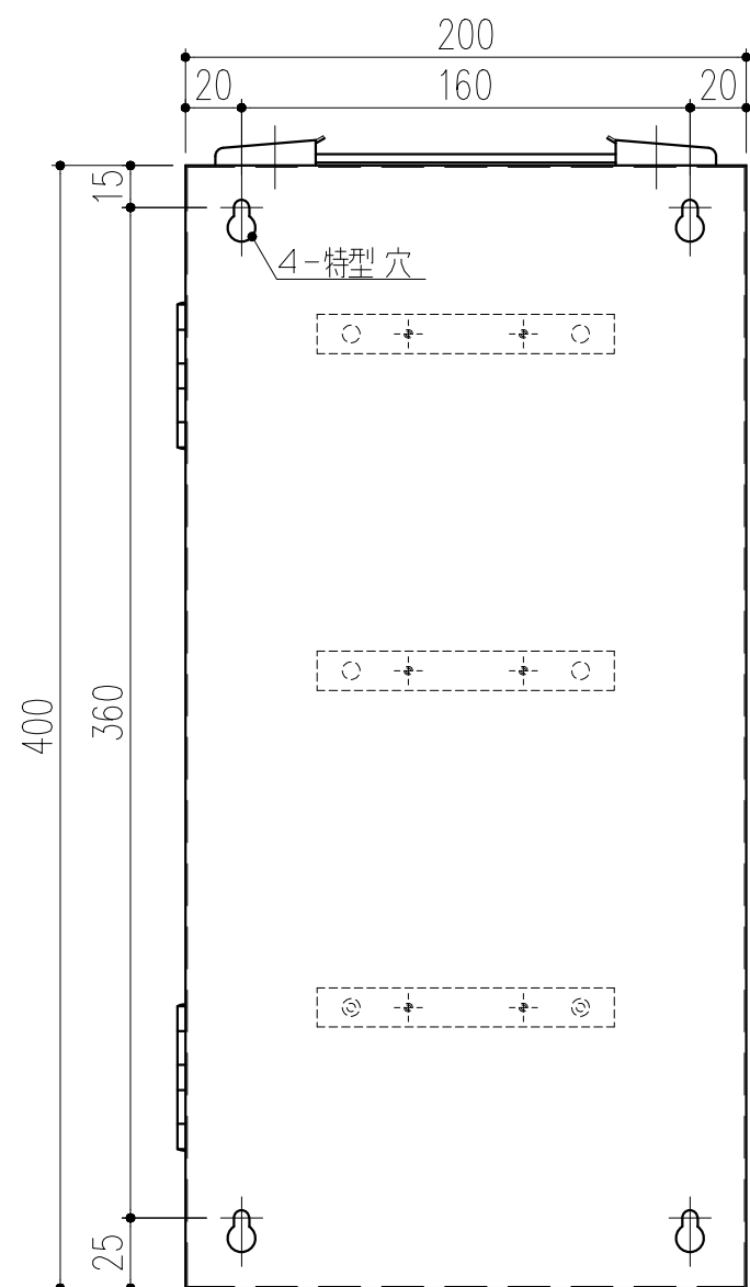
背面図 S=1/3
