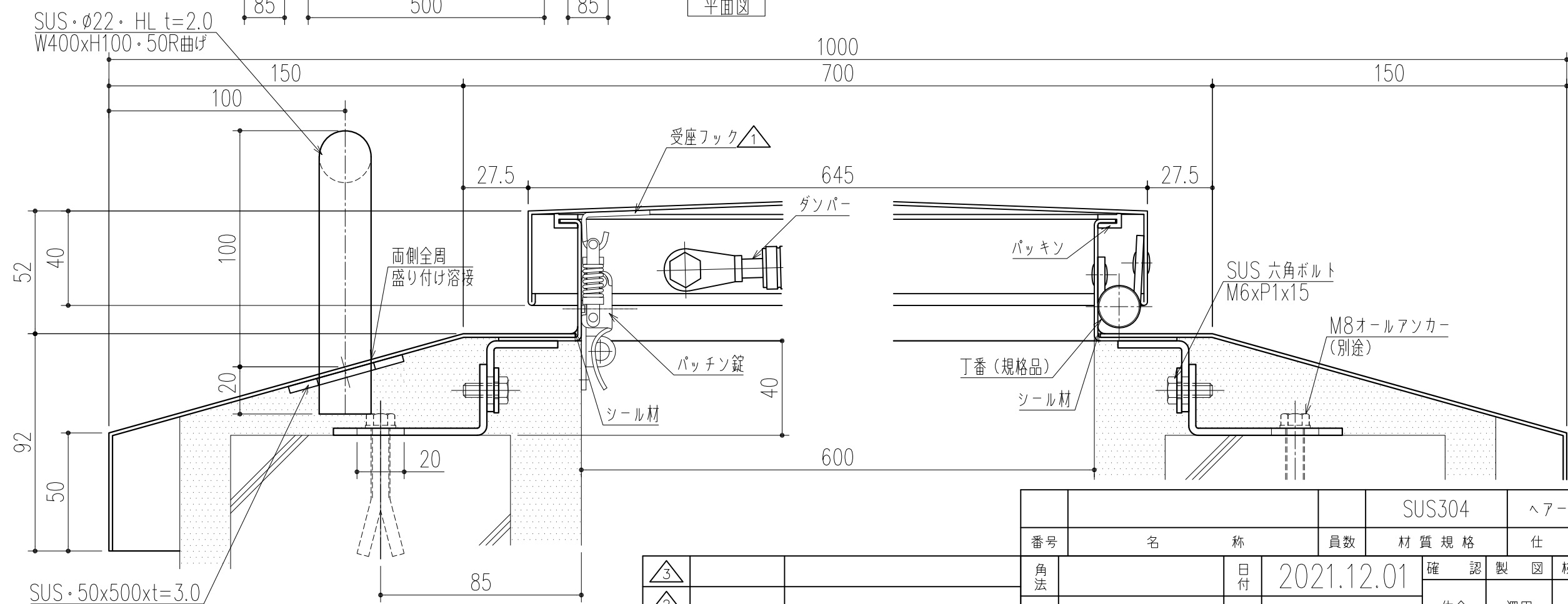
断面詳細図 S=1/2
