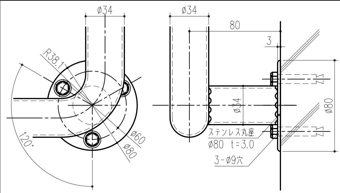
A部 取付詳細図 S=1/2
