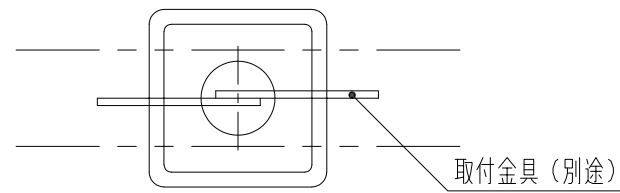
クサリ縦といの取付け例
