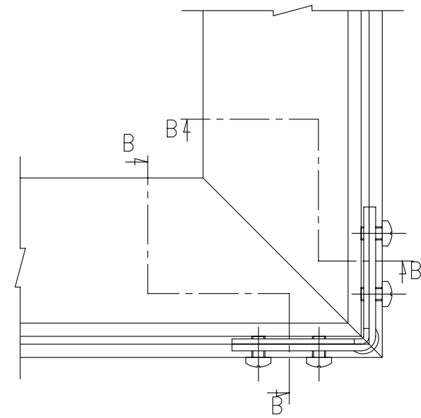
受枠との嵌合図 S=1:2
