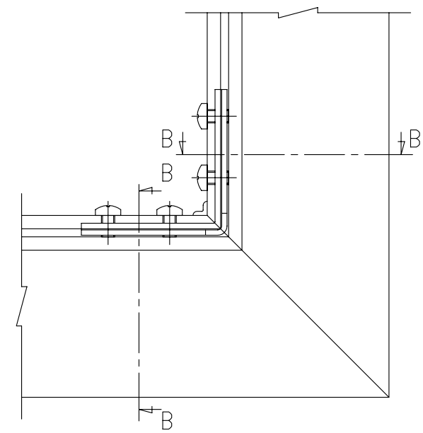
受枠との嵌合図 S=1:2
