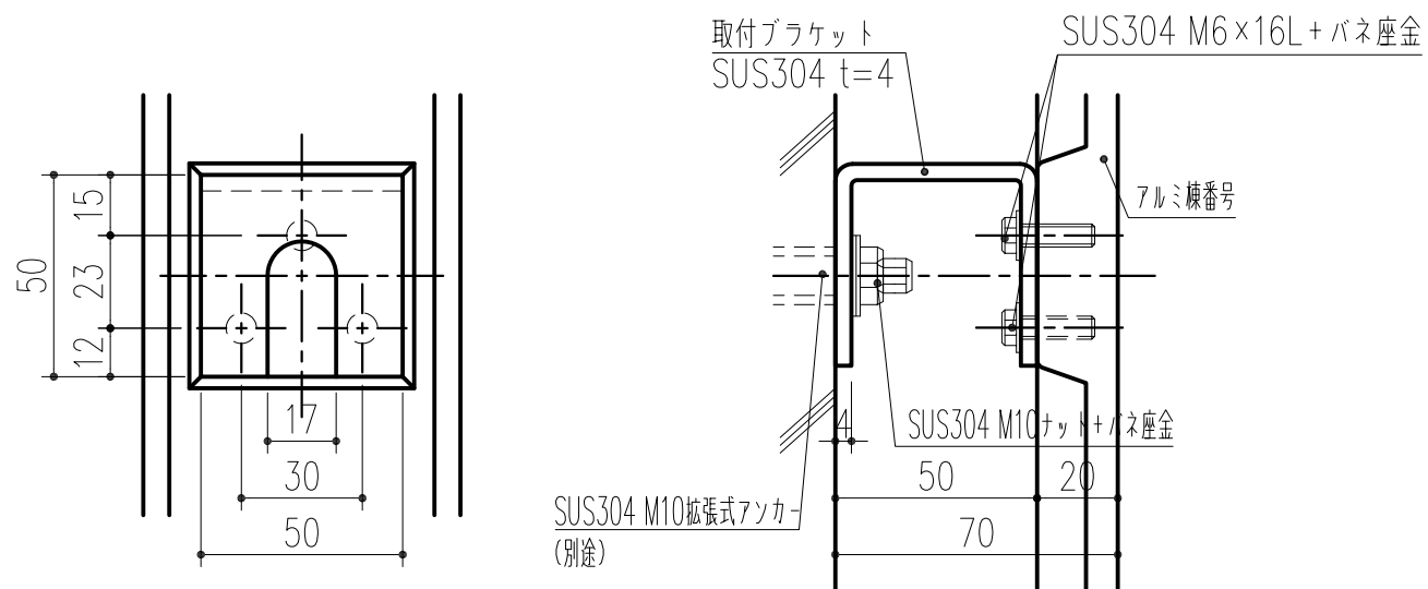
取付部分詳細図 S=1/2
