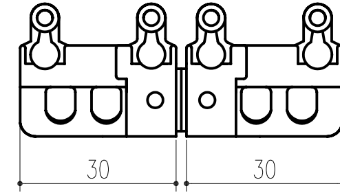
511-743 CFランナー-W S=1/1
