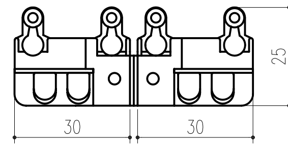
511-750 C後入れFランナー-W S=1/1
