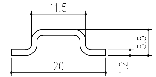
A部詳細図 1:2
