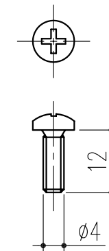
十字穴付なべ小ねじ M4×12 4本付属
