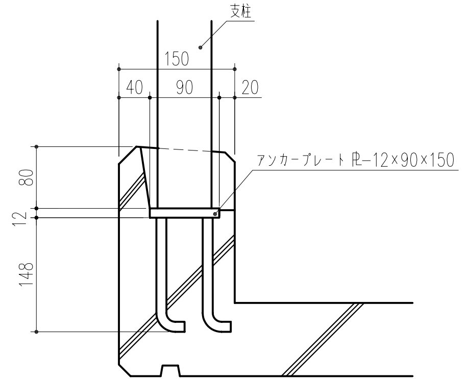
取付け例 1/5
