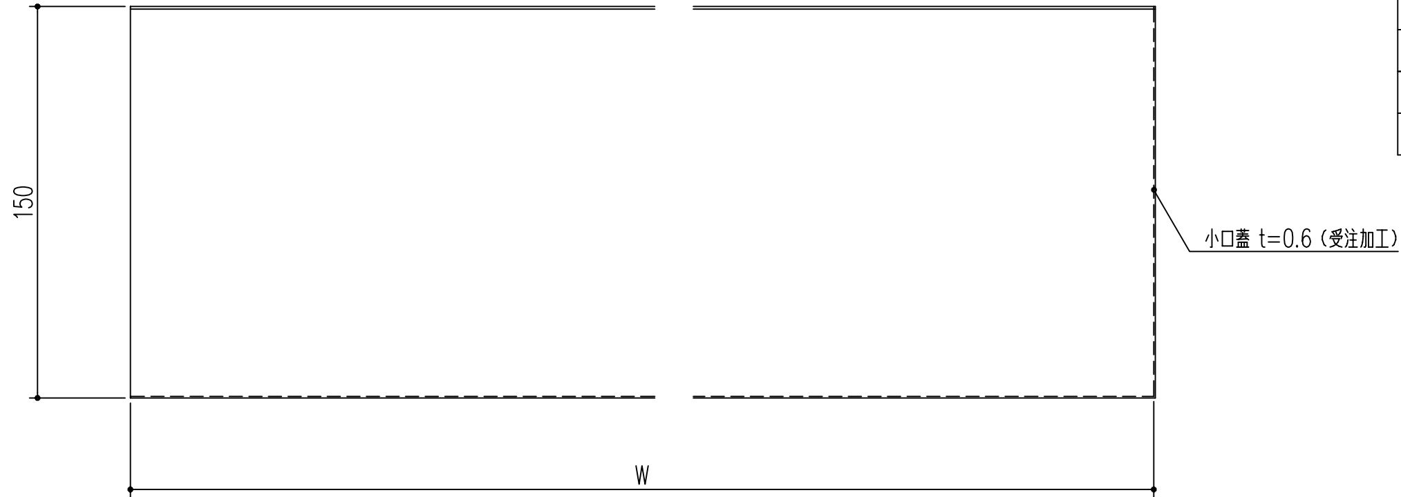
平面図
