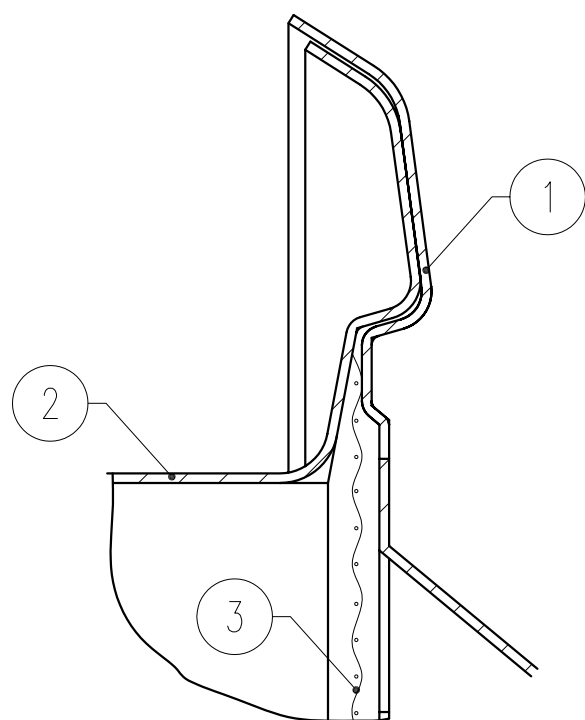
A部詳細図 S=2:1
