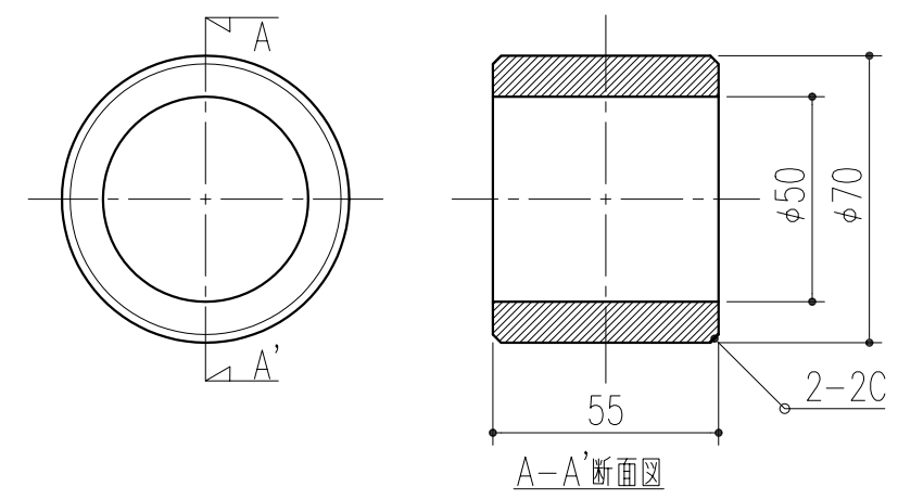
ゴムブッシュ詳細図
