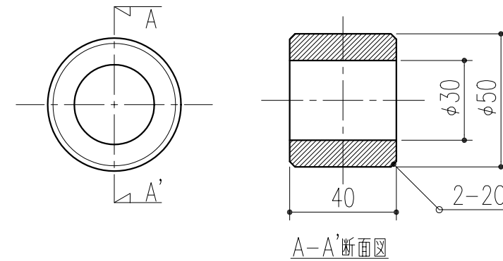
ゴムブッシュ詳細図
