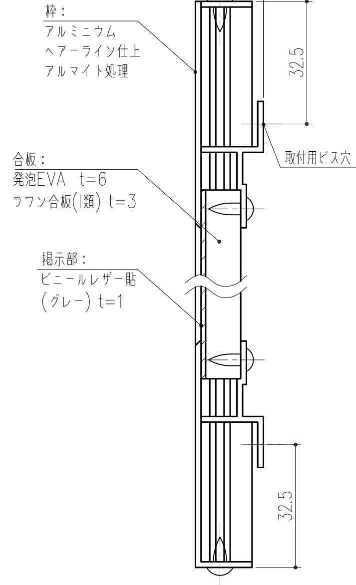
縦断面詳細図 S=1/1
