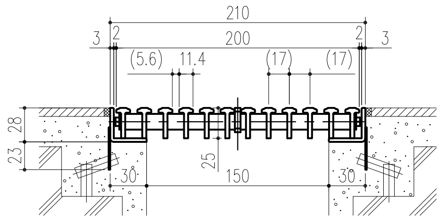
断面図
